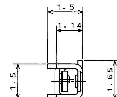
EXCEPT CRIMPPOT (クリンプ部を除く)
