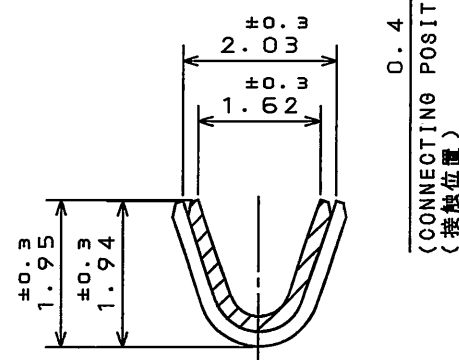
SECTION A-A (断面 A-A)
