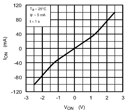
Fig. 13.1.4 I_{ON} - V_{ON}
