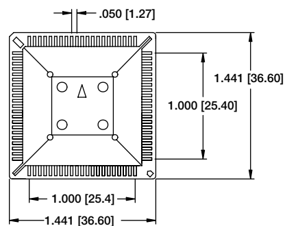
PLCC-84-AT
