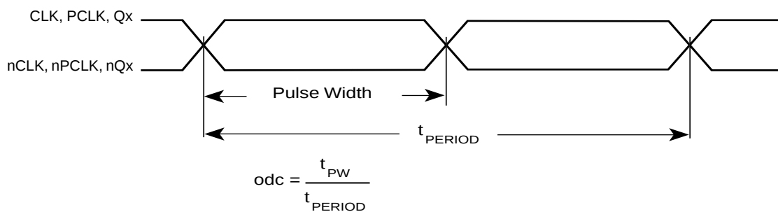
FIGURE 7 - odc & t_{PERIOD}
