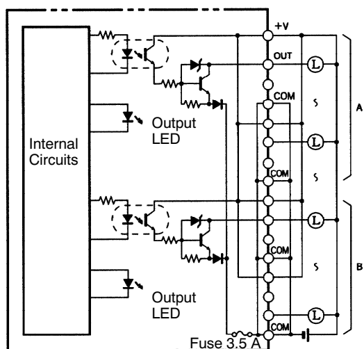
CQM1-OD213
