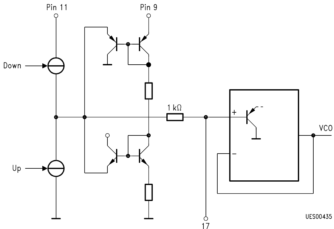
PLL-Filter (pin 17)
