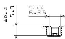
S E C T . B - B 断面 B - B ( S C A L E 1 : 1 )
