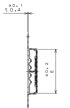
S E C T I O N C - C 断面 C - C ( S C A L E 1 : 1 )
