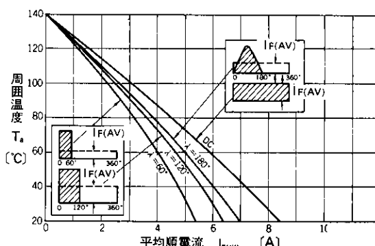
平均順電流—周囲温度 (冷却体AC01-5B) 自冷
