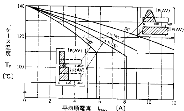
平均順電流—ケース温度
