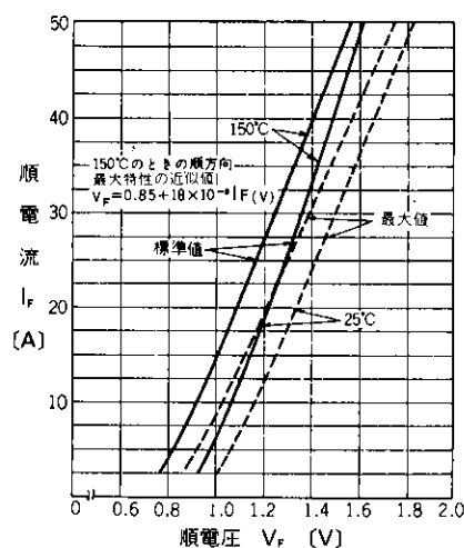
順特性
