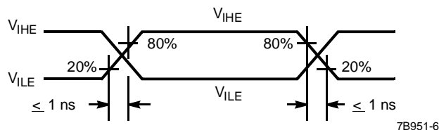
(d) ECL Input Test Waveform
