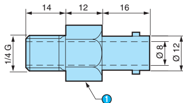
Sub-base : 79 696 041
