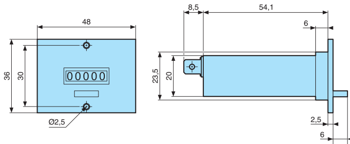
99 766 71 : 36 x 48 - 5 decades
