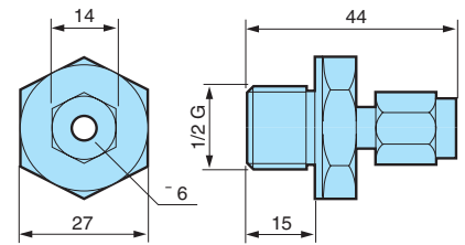
Connection : 79 696 040
