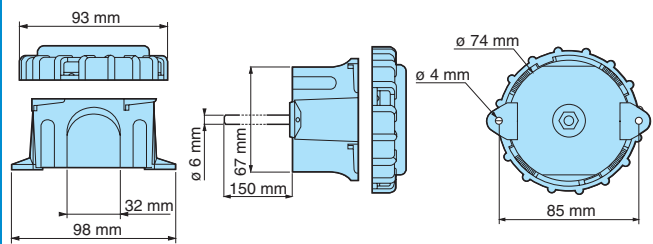
89 750 151
