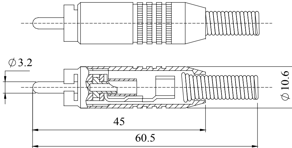
Dimensions
