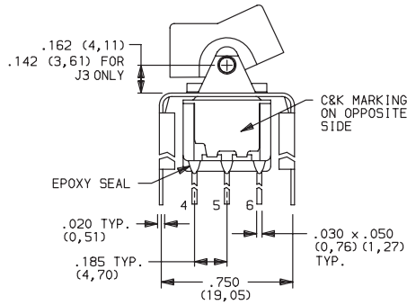
7201J1_BE2 DPDT
