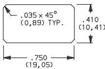
J11 & J21 Actuators
