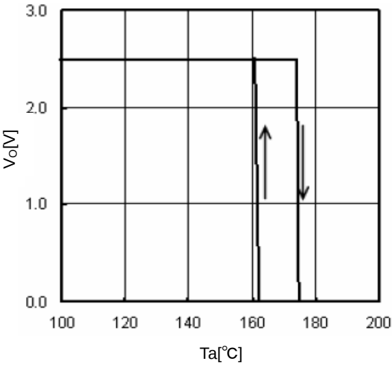
Figure 28. TSD
