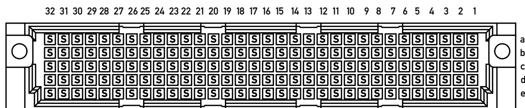
Bestückungsplan / contact layout
