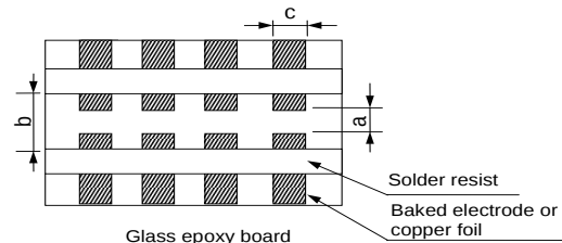
Fig.3 (in:mm)
