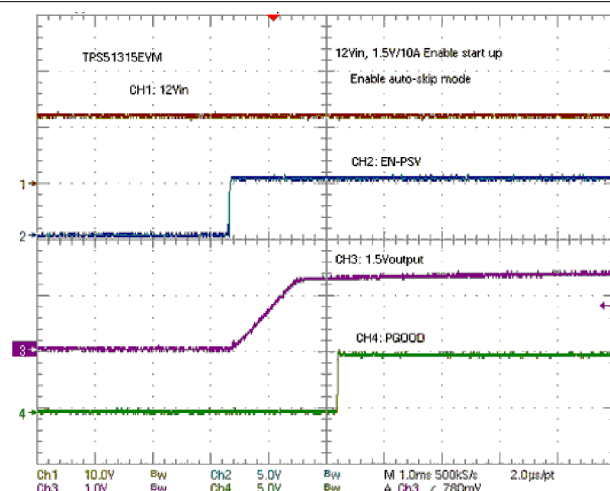
Figure 9-7. Enable Turn-On
