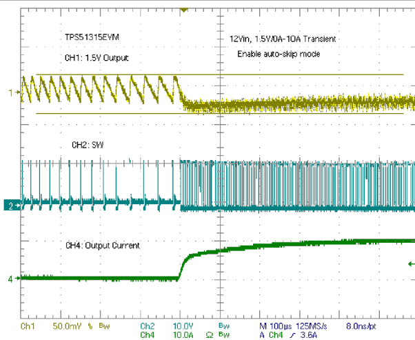
Figure 9-3. 0-A to 10-A Load Transient Rise
