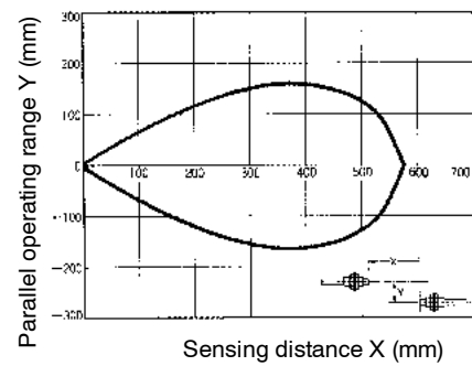
E32-T61 with E3X-NH amplifier
