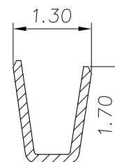
SEC A-A
