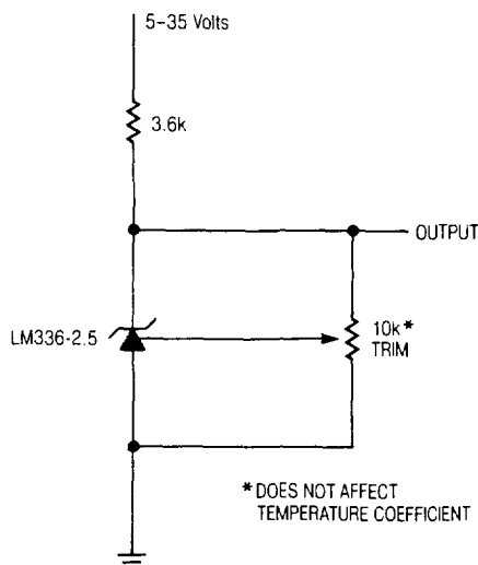
2.5 Volt Reference
