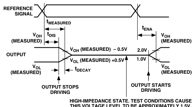
Figure 27. Output Enable/Disable
