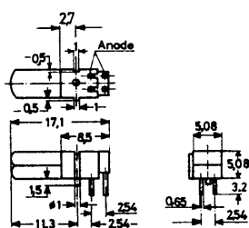
Einbaulage Mounting Position
