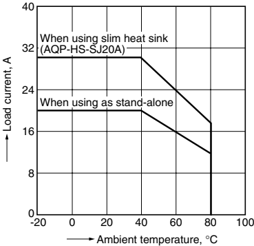
(1) 30A type (AQAD511DL)
