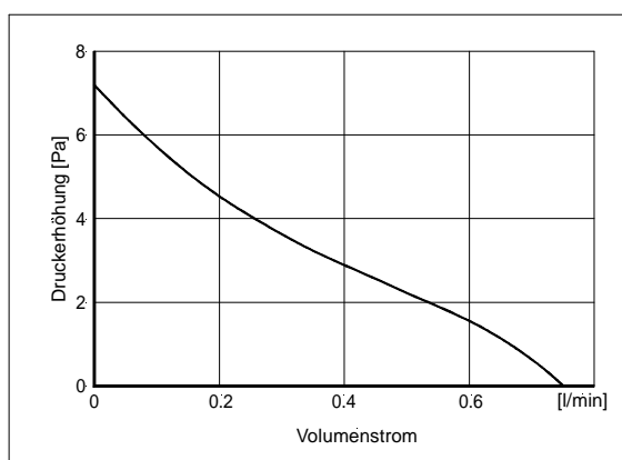
LÜFTERKENNLINIE
