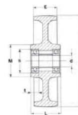
CUSCINETTO A RULLINI STANDARD O INOX - STANDARD OR STAINLESS STEEL ROLLER BEARING - STANDARD ODER ROSTFREIES ROLLENKORBLAGER - ROUEMENT À ROULEAUX STANDARD OU INOX - COJINETE A RODILLOS STANDARD O INOX
