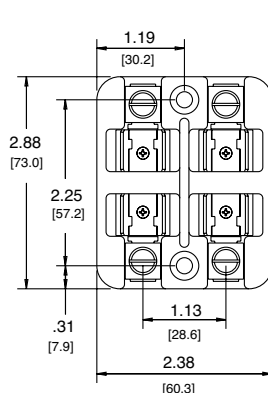
2 POLE
