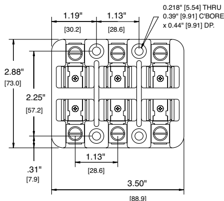
3 POLE
