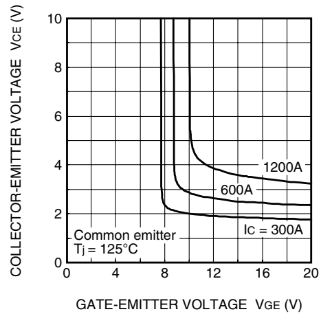
V CE - V GE
