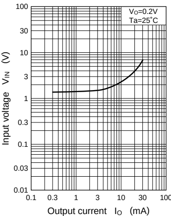
V_{IN} - I_O
