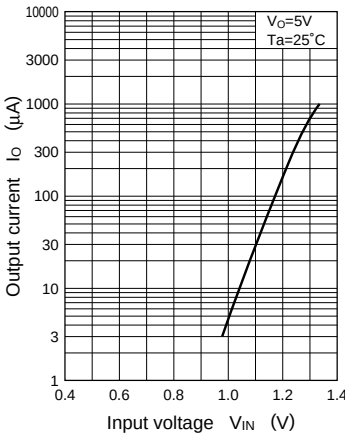
I_O - V_{IN}
