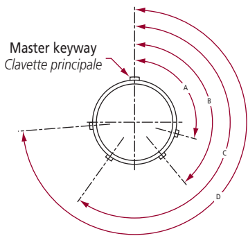
Plug front view / Fiche, vue face avant
