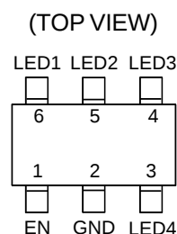
SOT-23-6
