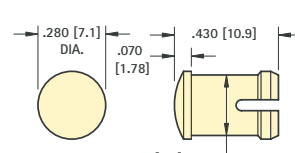
FIG. 4 T-1 3/4
