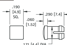
FIG. 6 T-1
