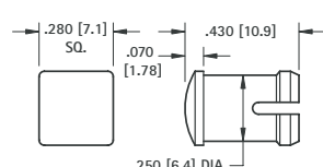
FIG. 7 T-1 3/4
