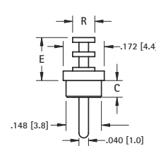
Feed-Thru
