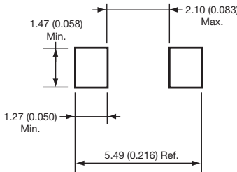
DO-214AC (SMA)
