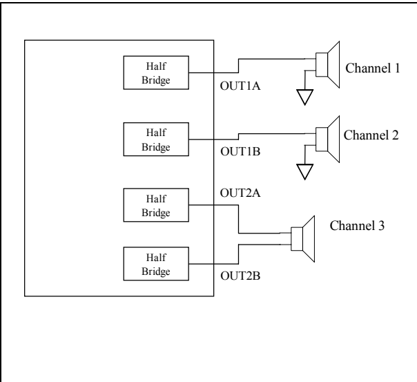
Figure 30. OCFG = 01
