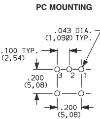
TS01ABE Horizontal Actuation SPDT
