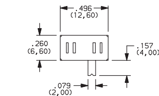
Actuator shown in pos. 3
