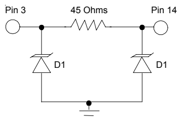
CLK
