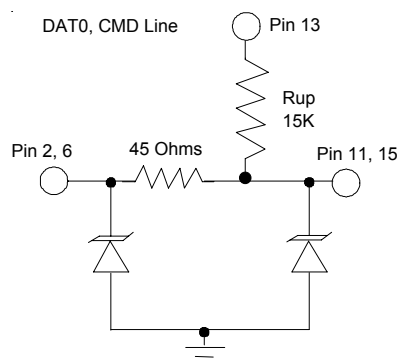
DAT0, CMD
