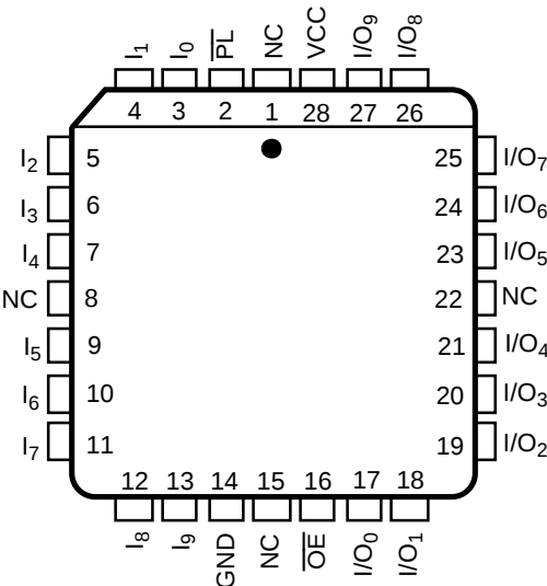
PLCC JEDEC
