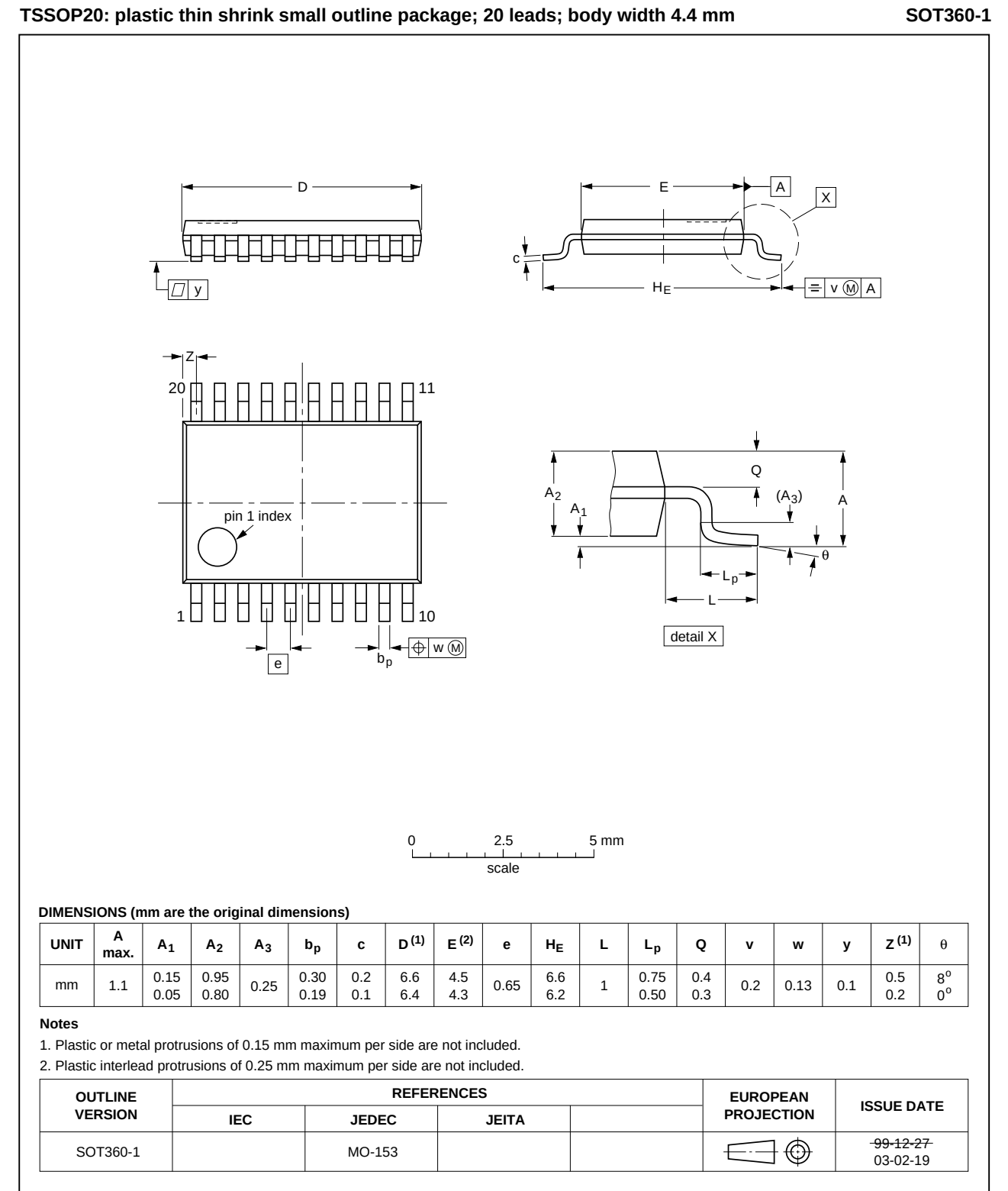
Fig 14. Package outline SOT360-1 (TSSOP20)
