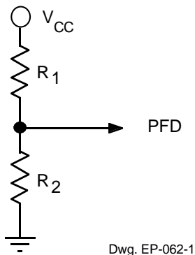
Dwg. EP-062-1
