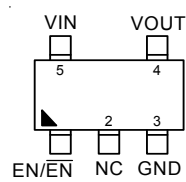
TSOT-23-5/SOT-23-5/ SC-70-5
