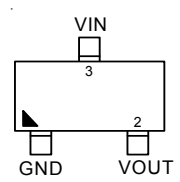
TSOT-23-3/ SOT-23-3
