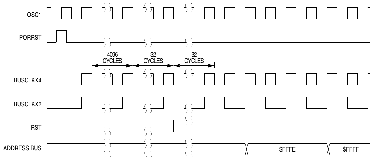
Figure 13-6. POR Recovery
