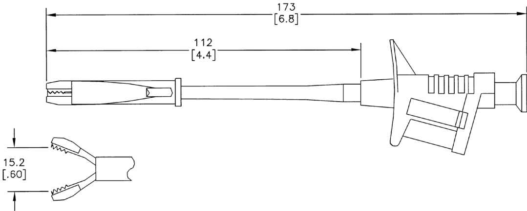
Dimensions : Millimetres (Inches)
