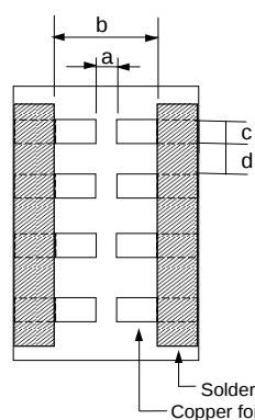
Fig. 3 (in:mm)
