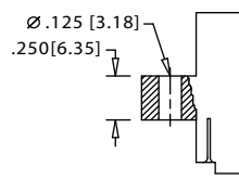
FLUSH MOUNTING (D)
