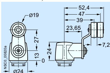
Schwenkhebel, 2 Rollen 19 mm
