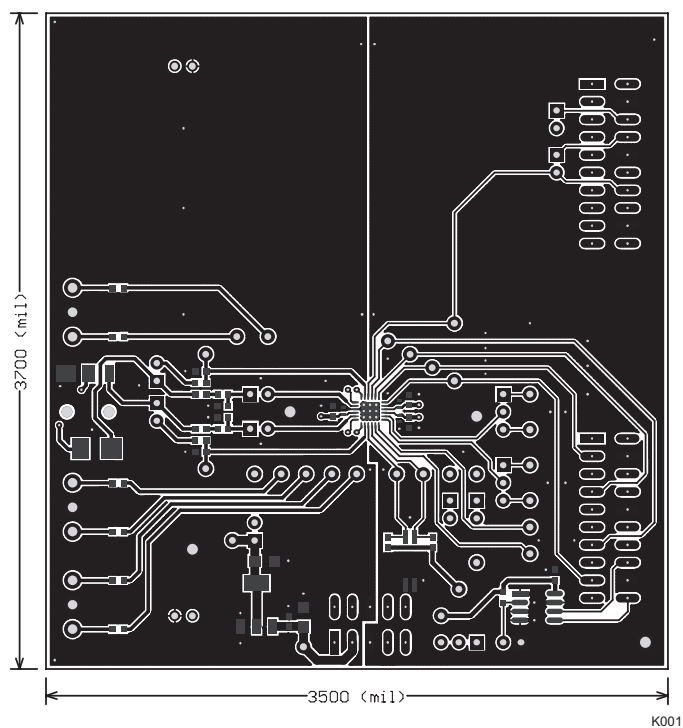
Figure 20. Top Layer
