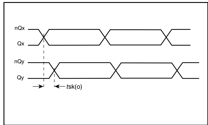
Output Skew
