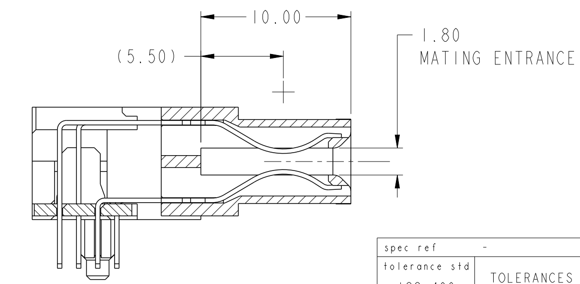
SECTION D-D
