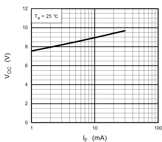
Fig. 12.4 V_{OC} - I_F
