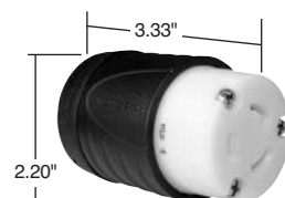
20A Connector
