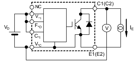
Fig. 2 V_{EC} Test
