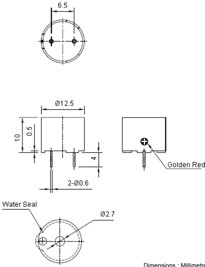
Dimensions : Millimetres
